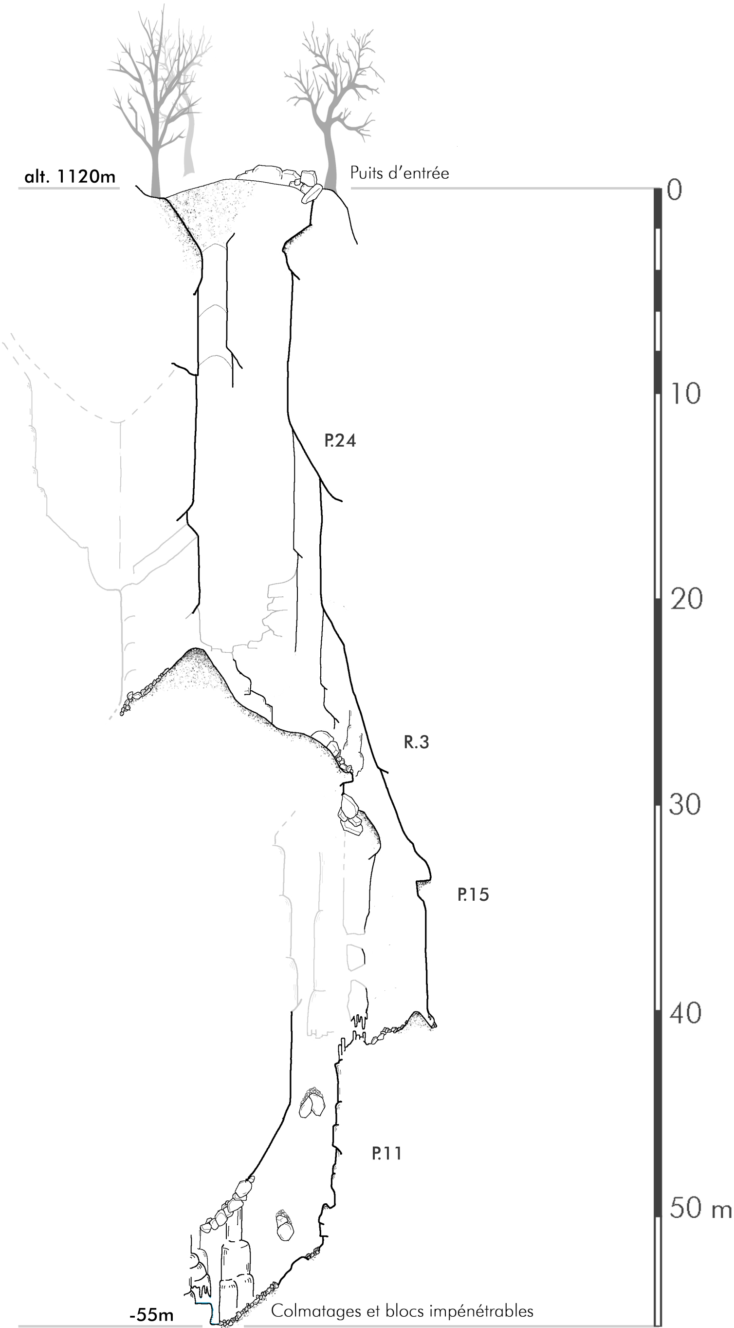
Coupe Développée
